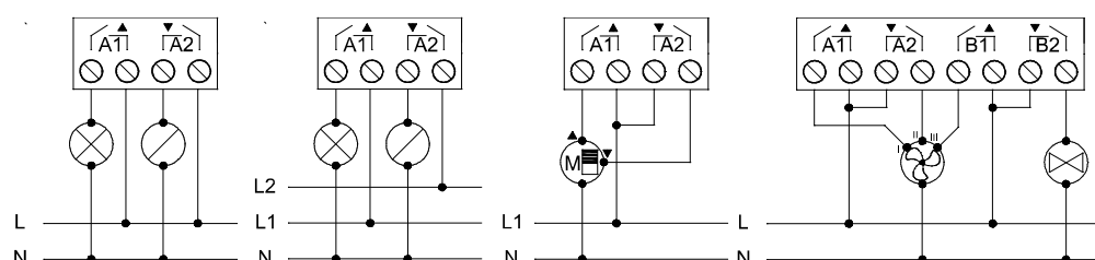
Figure 3. Exemples de connexions (de gauche à droite): 2 charges, 2 charges a phases différentes, volet roulant et ventilo convecteur
